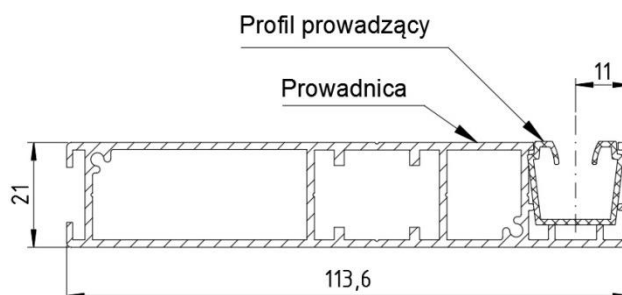
Rys. 9. Prowadnicą do systemu z kasetą podtynkową – elementy.
