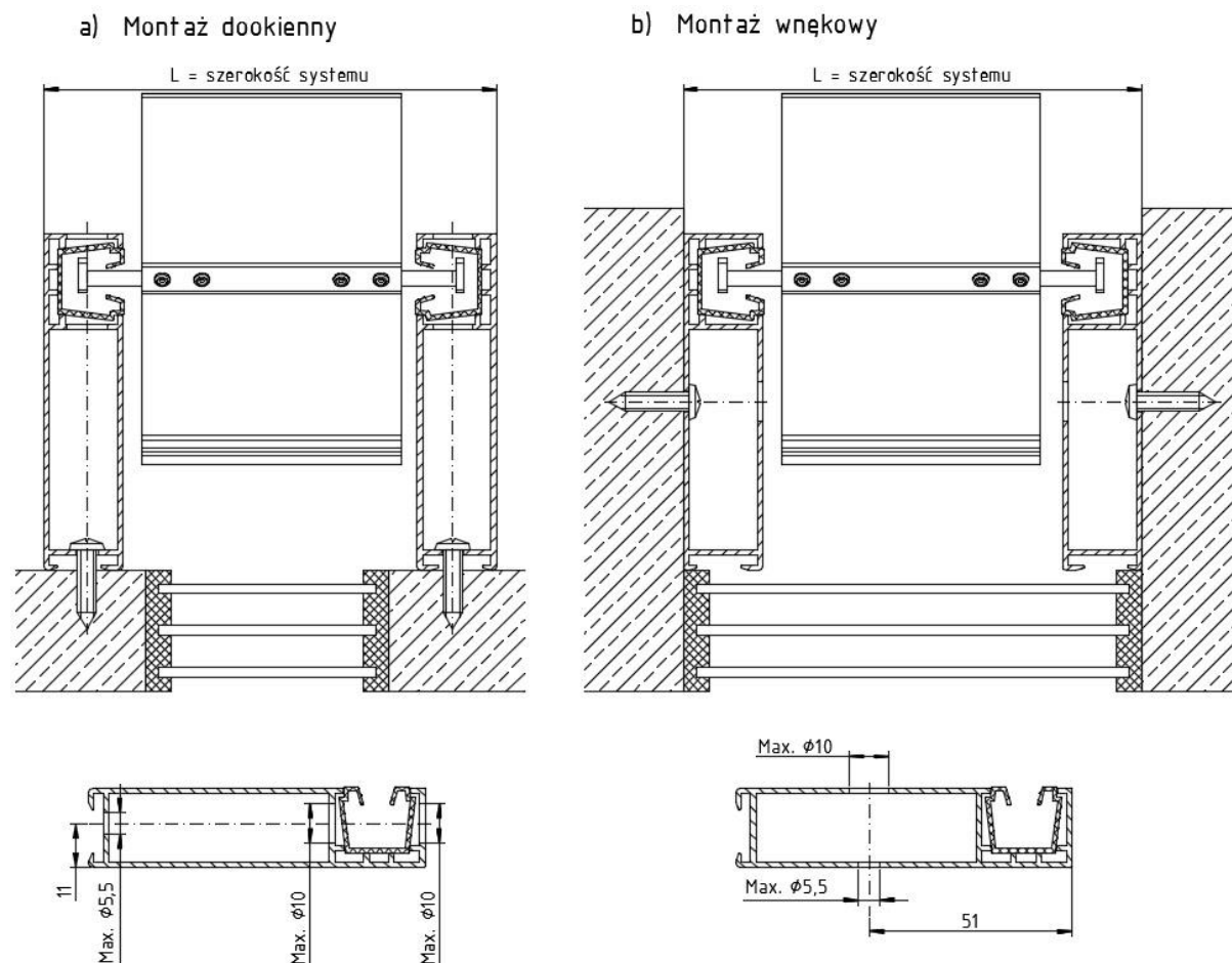
Rys. 6. Sposoby montażu prowadnicy dookiejnej: a) – Montaż dookiejny b) - Montaż wewnętrzny
