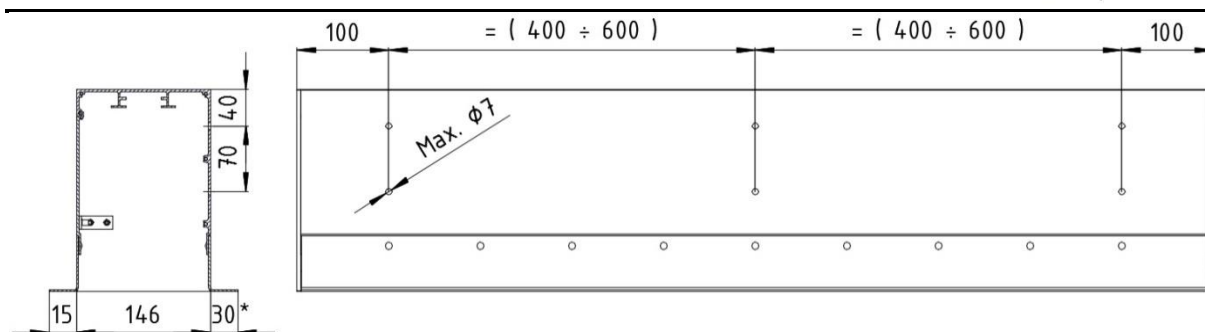
Rys. 13. Schemat wykonywania otworów montażowych w kasie podtynkowej. * - Wymiar zmienny, standardowo 30 mm.
