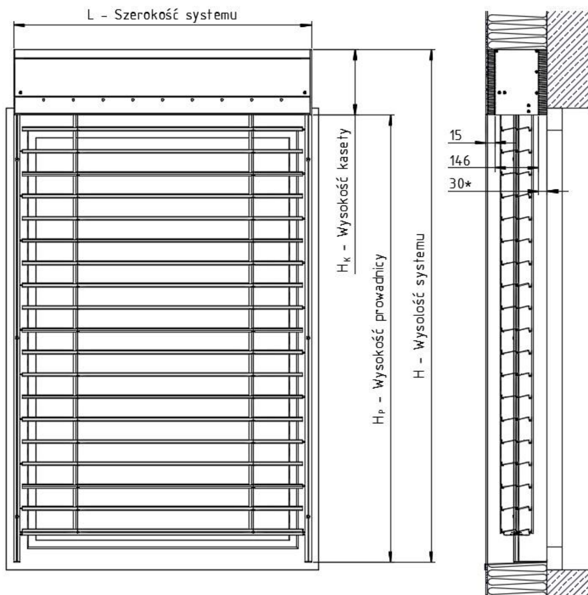
Rys. 11. Wymiary systemu żaluzji fasadowych Z90 z kasetą podtynkową. * - Wymiar zmienny, standardowo 30 mm.
