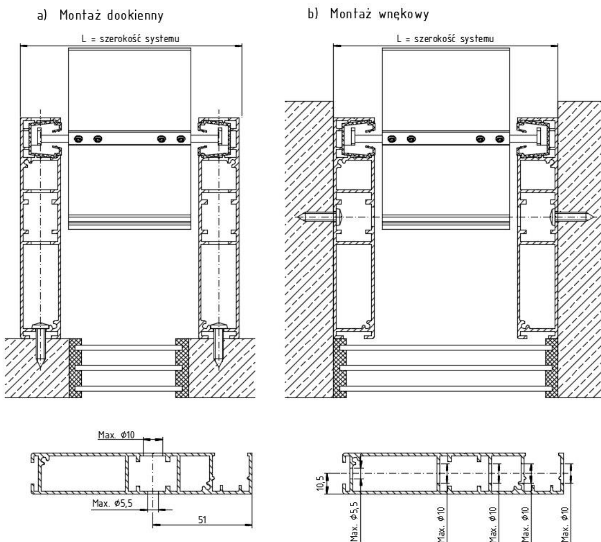
Rys. 12. Sposoby montażu prowadnicy: a) – Montaż dookienny b) - Montaż wnąkowy
